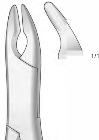
CRYER DD-10070 Fig. 150A
