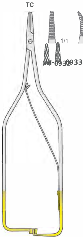
ARFUGA DD-0937 160 mm
